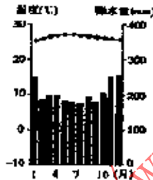
新加坡气温曲线和降水柱状图
