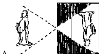
小孔成像
