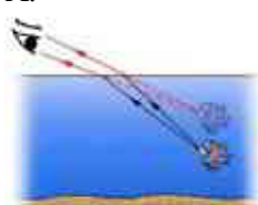
水中的鱼看起来变浅了
