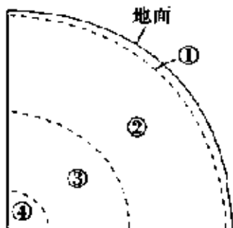
地球的内部圈层结构
