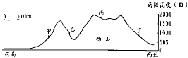
图1 北京西山地形剖面示意图
